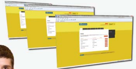
Parklahalduri kasutusliides
